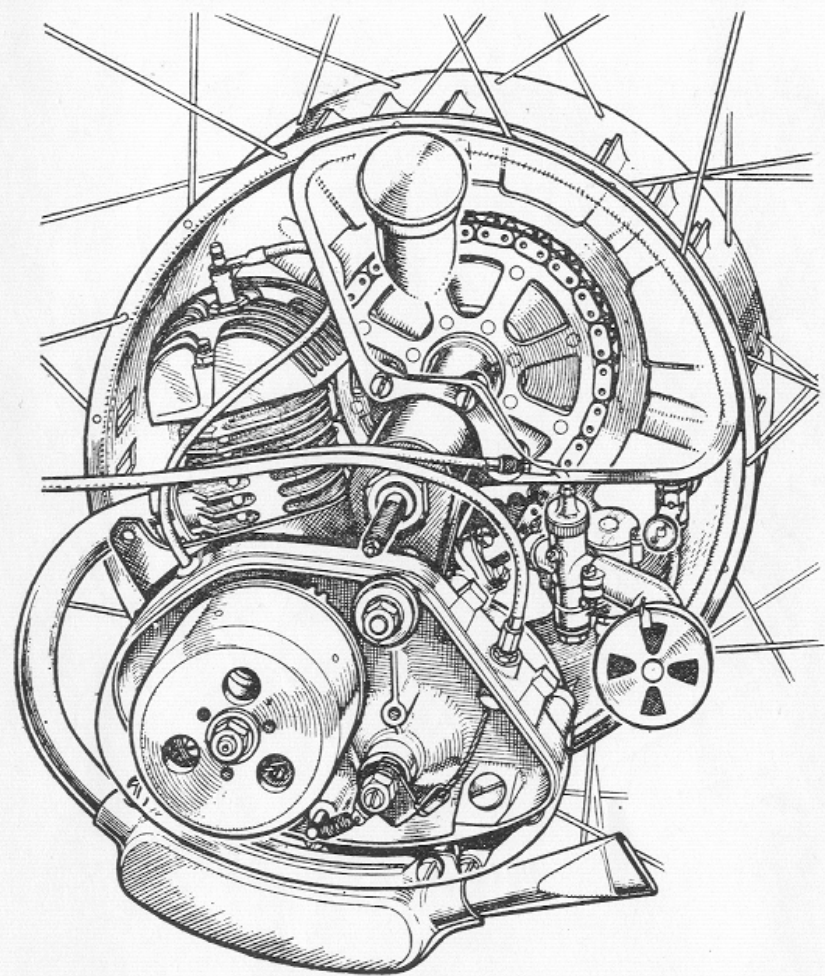
Den kända Cyclemaster genom röntgenögon
