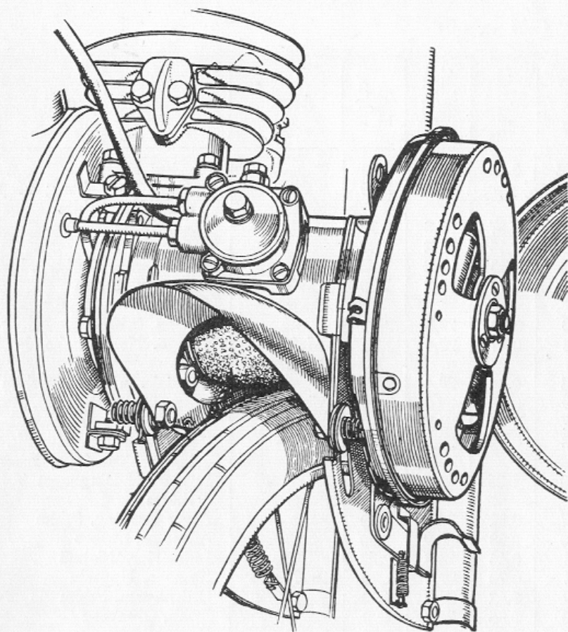
Velosolex med drivrulle
